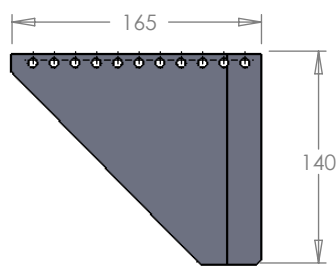
2- & 4-+ Fin Aluminium 90 deg. 0030A (Standard)
