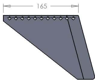
2- & 4-+ Fin Aluminium 0030AA (Avon Type)
